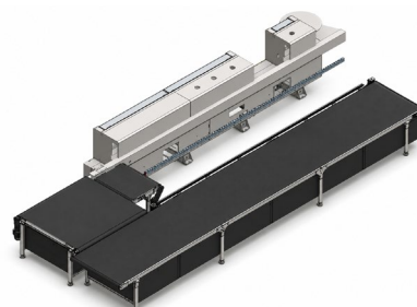
ESTEIRA DE RETORNO EDGE 8 TURBO
